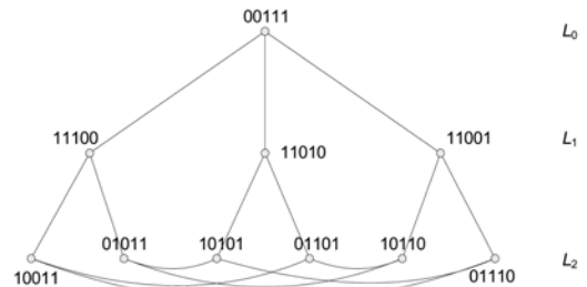
그림 1 유사 계층 연결망으로 나타낸 O_3
