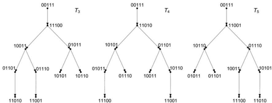
그림 2 O_3 의 에지 중복 없는 스페닝 트리들
